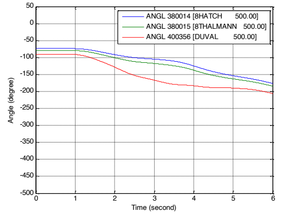
(d) 45%PV +15%WT
