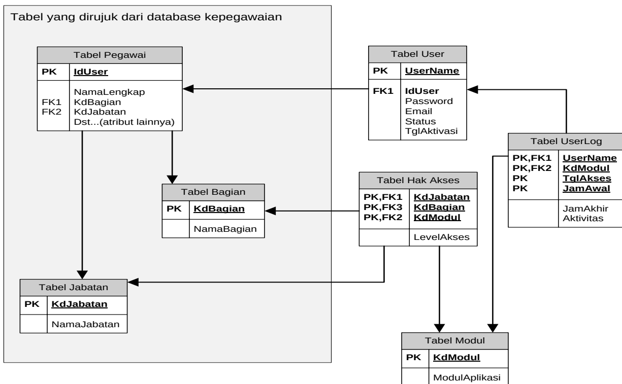
Gambar 12. Desain database
