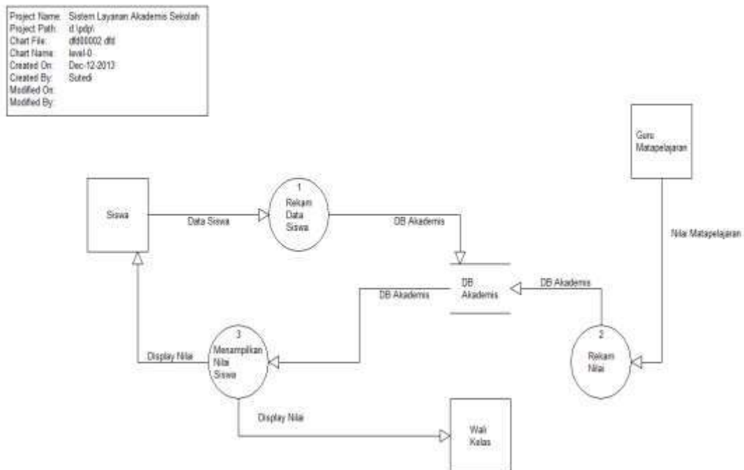
Gambar 7. DFD Level-0
