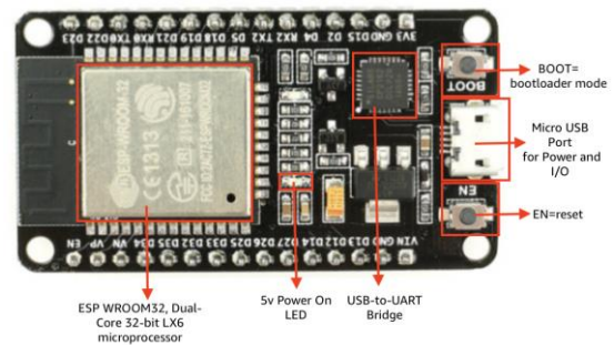
Figure 6. ESP32 DEVKIT V1
