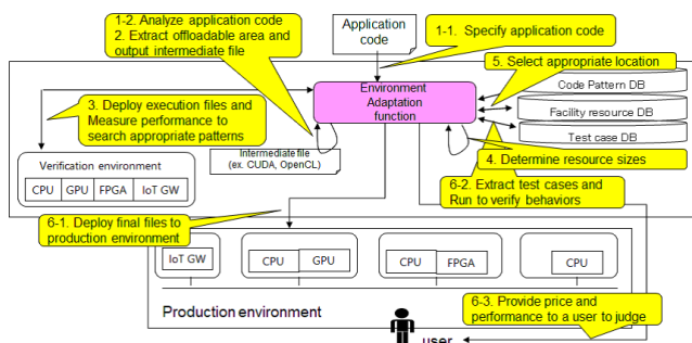
図 1 環境適応ソフトウェアの処理ステップ
