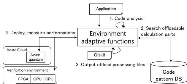
図 2 量子コンピュータへのオフロード処理
