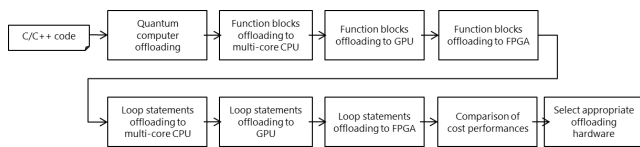
図 2 混在環境への適切な自動オフロード方式
