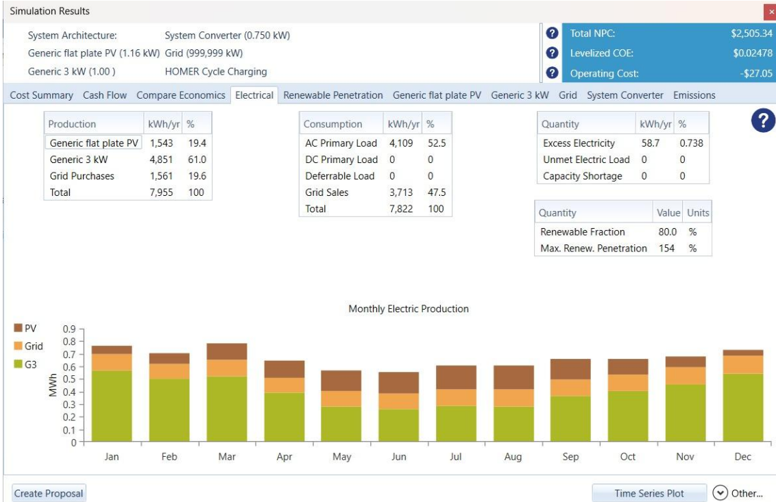
Şekil 2. Üretilen Elektrik Miktarı
