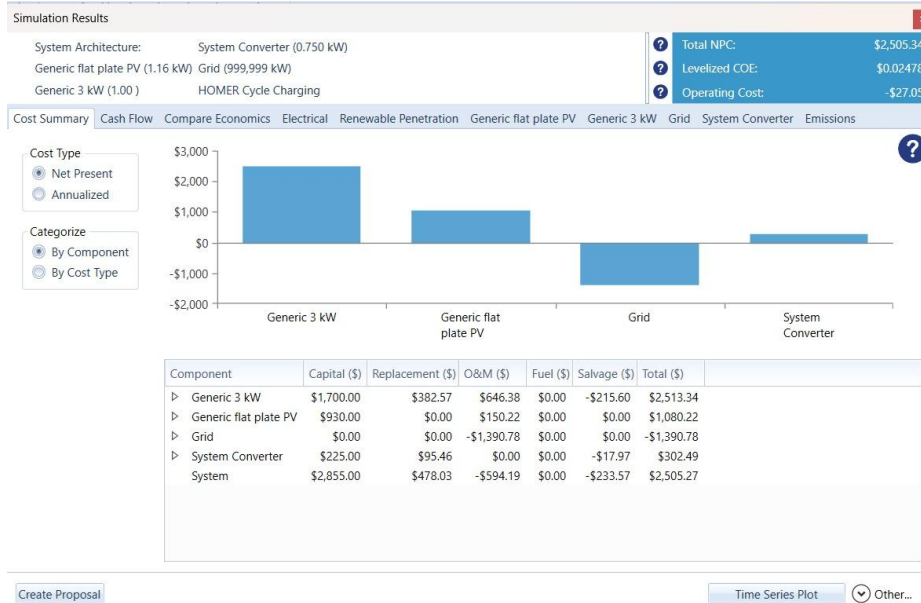
Şekil 5. Sistemin Maliyet Grafiği
